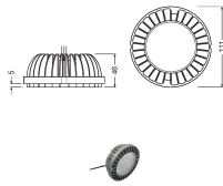
Technische Daten Osram PrevaLED Coin MR16 G2 12W 1200lm 40D - 840
