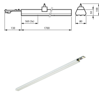
Technische Daten Philips LED Tragschiene Coreline LL217X 49W 8000lm 35x71D - 840 | 1700mm - 5-polig
